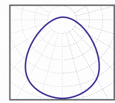
косинусная КСС 90°
