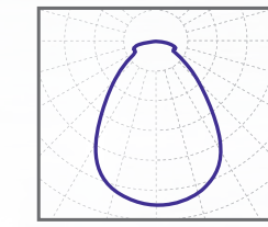
косинусная КСС 80°
